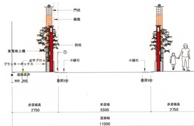
■道路横断面図
