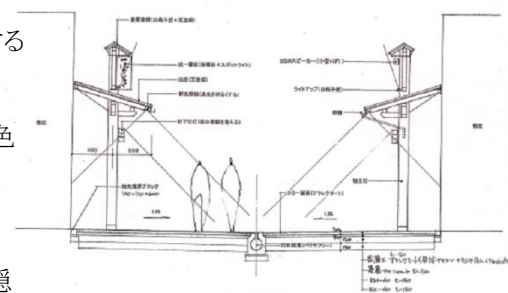
■道路横断面図
