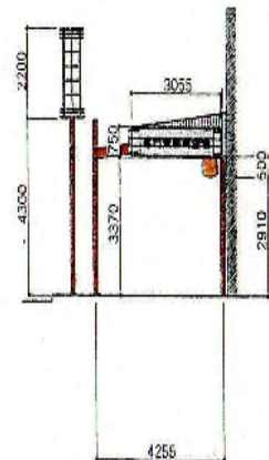
■アーケード断面図
