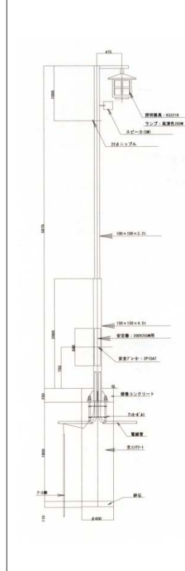
■図6 街路灯
