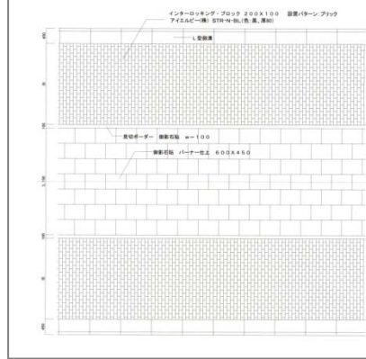
■図5 道路舗装
