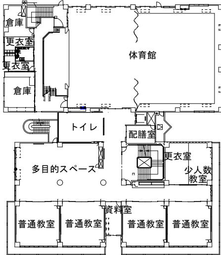
4階平面図
