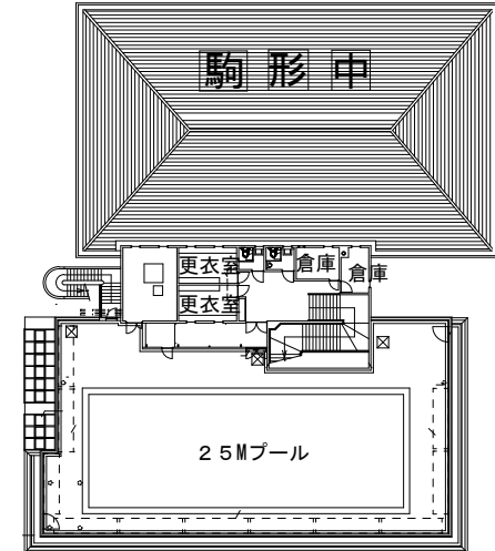
6階平面図
