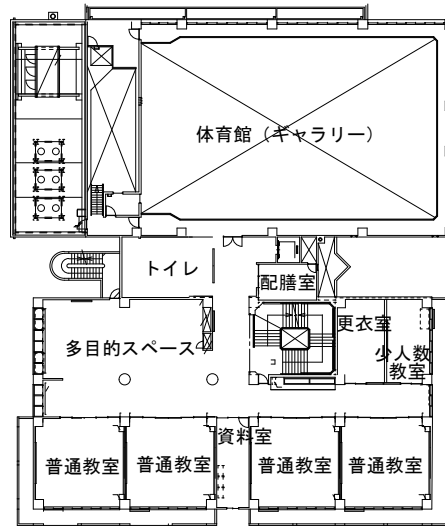
5階平面図
