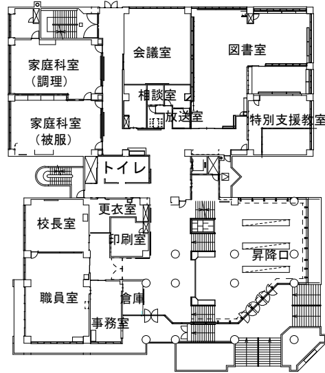
2階平面図
