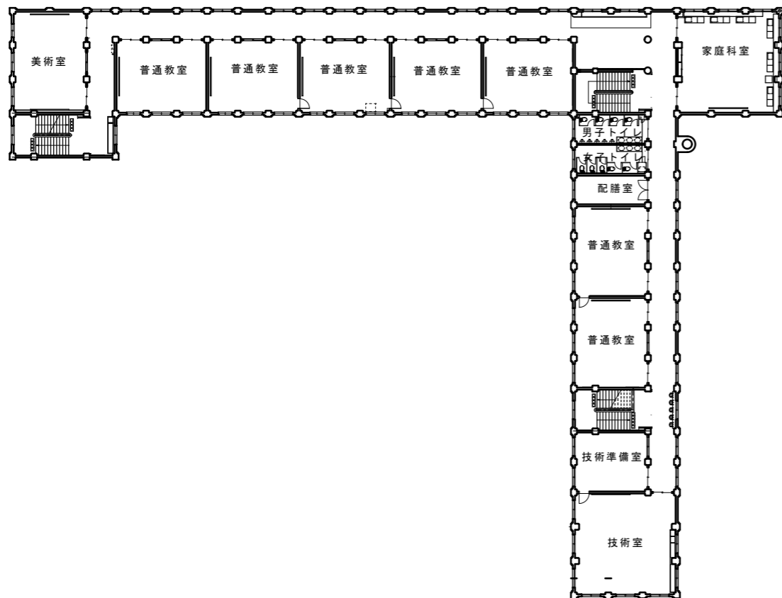
3階平面図
