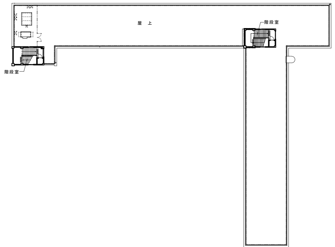
塔屋階平面図
