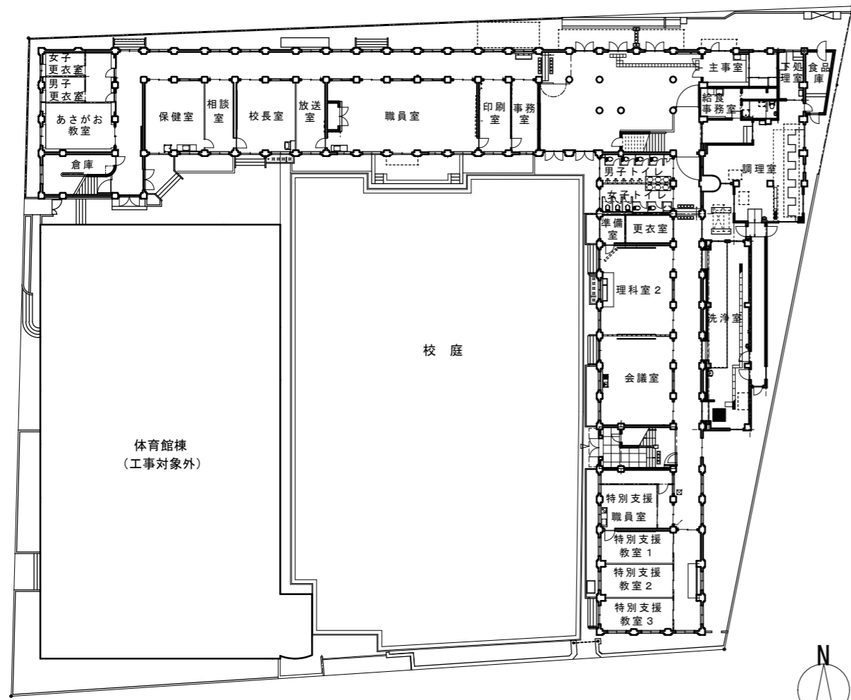
1階平面図
