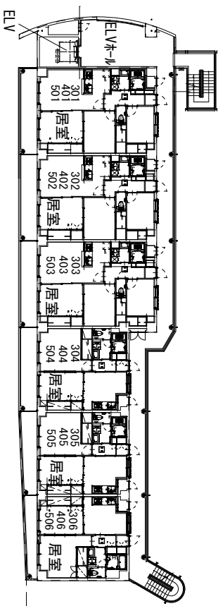
3～5階 平面図
